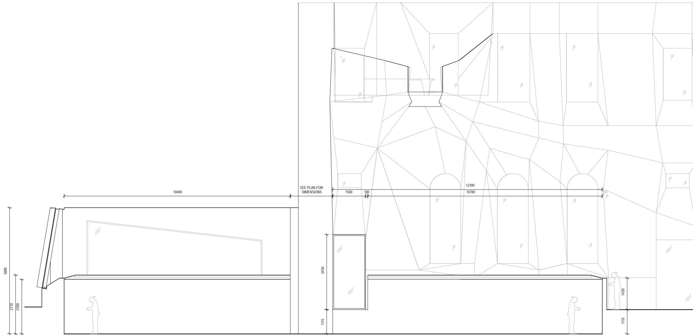
Elevation A
